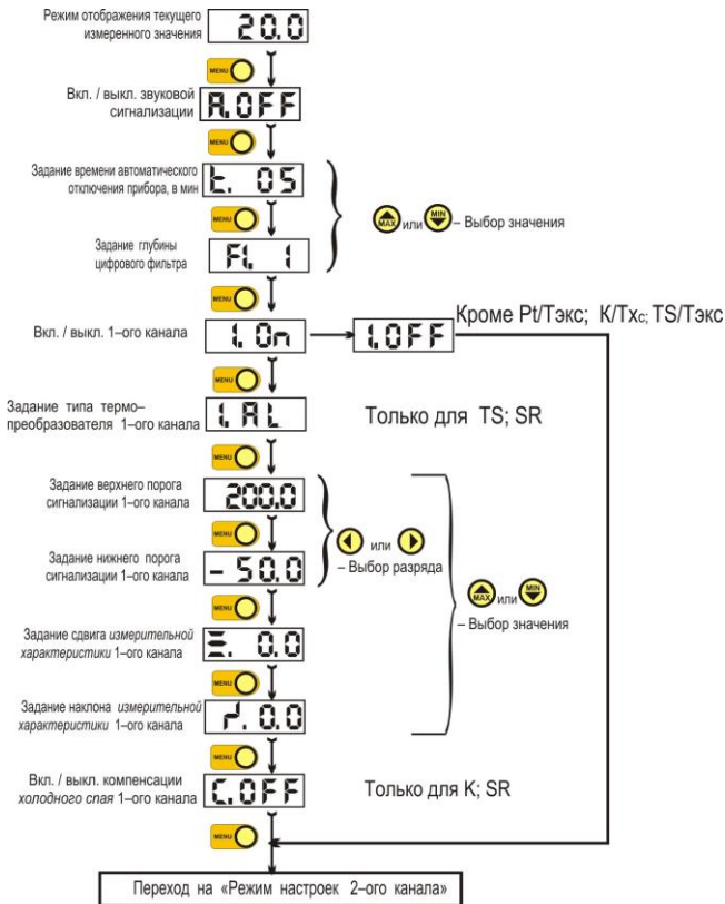
Рисунок 3 – Алгоритм режима настроек прибора PT-8 (Общие настройки и настройки 1-ого канала)
