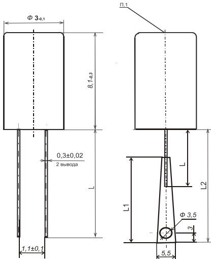
Реле с проволочными выводами
