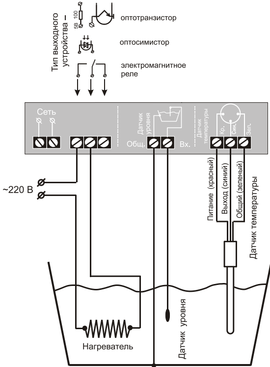
Схема электрическая подключения регулятора температуры РАТАР-02.п/п-D1
