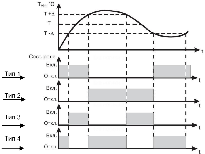
Рисунок 3 – Диаграммы работы выходного устройства регулятора температуры РАТАР-02.п/п
