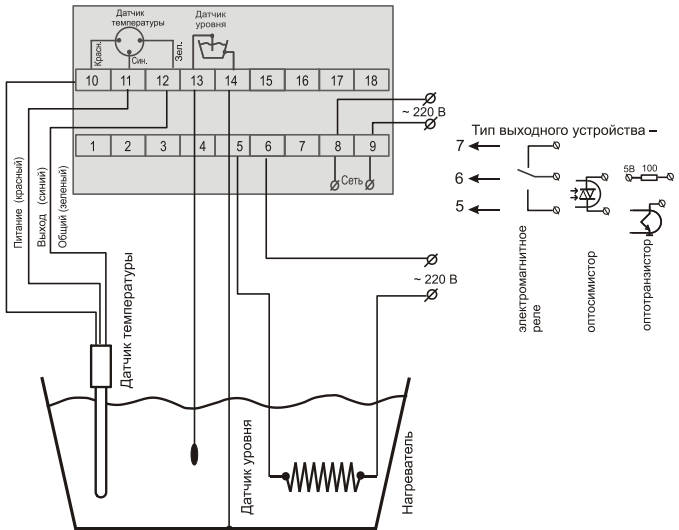
Схема электрическая подключения регулятора температуры RATAР-02.п/п – Щ1
