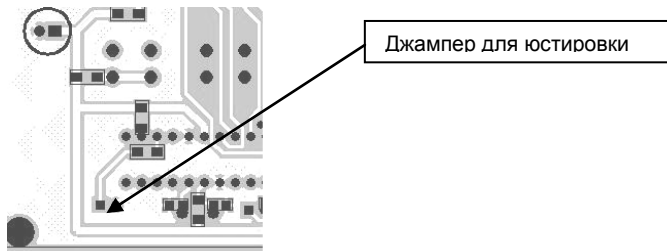
Регулятор температуры РАТАР-02.п/п-Н2
