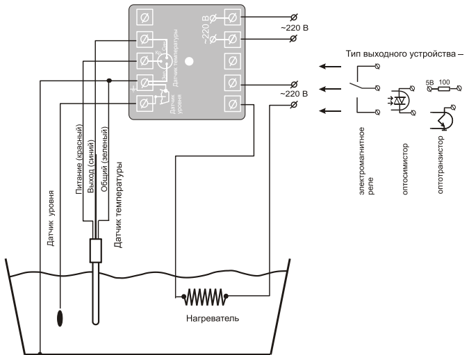
Схема электрическая подключения регулятора температуры РАТАР-02.п/п – ЩЗ
