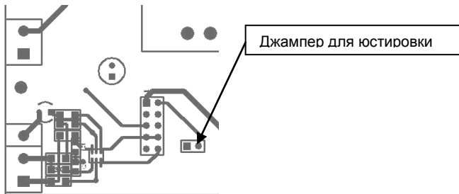
Регулятор температуры РАТАР–02.п/п–D1
