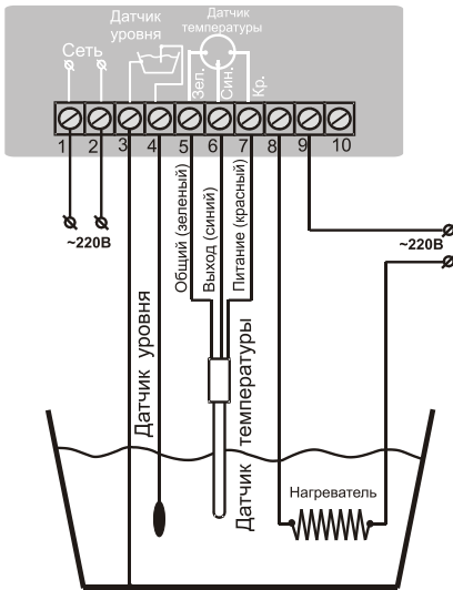
Схема электрическая подключения регулятора температуры РАТАР-02.п/п-Н2
