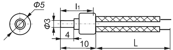
Рисунок 1 – Термопреобразователи сопротивления ТСPr и ТСMг в конструктивном исполнении K0
