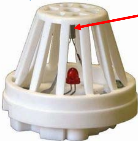
Малогабаритный пожарный извещатель ИП103-4/1-А2 «МАК-1»
