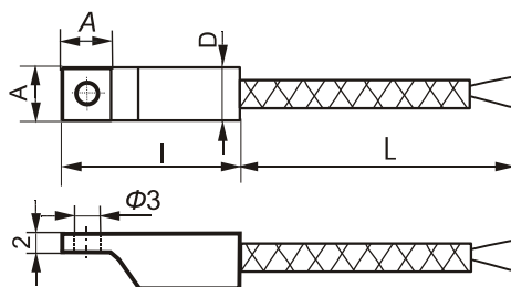
Рисунок 1 – Термопреобразователи сопротивления ТСPr и TCMr в конструктивном исполнении K5
