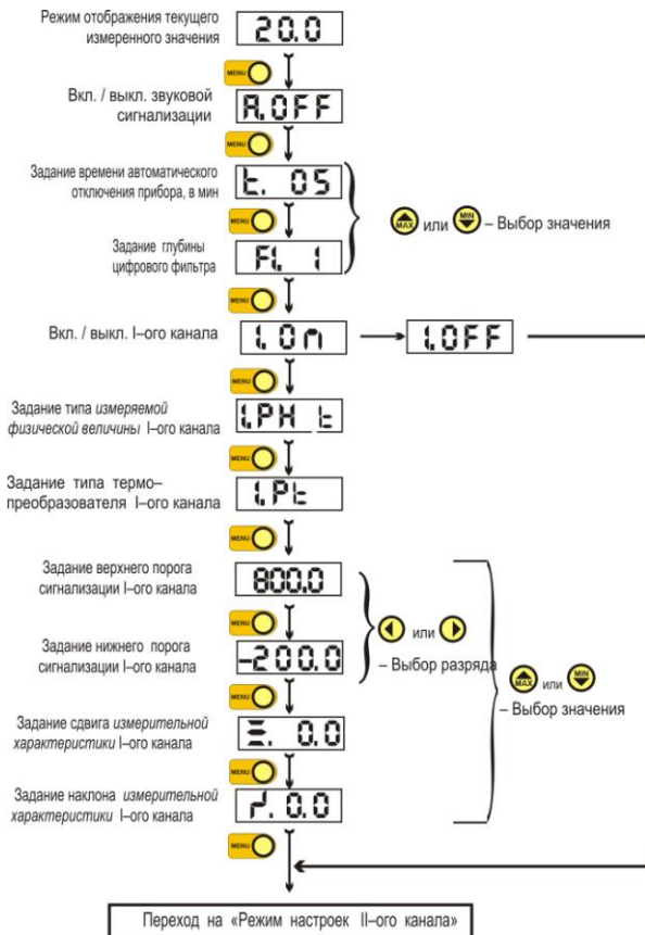
(Параметры физических величин показаны условно) Рисунок 3 – Алгоритм режима настроек мультиметра IT-8-RUT (Общие настройки и настройки I-ого канала)
