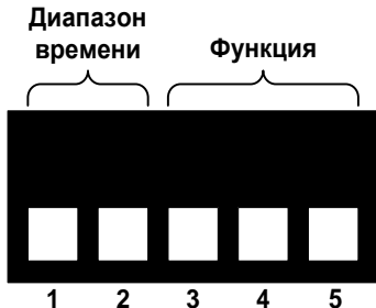
Рисунок 2 – Расположение переключателей реле времени РВ-01
