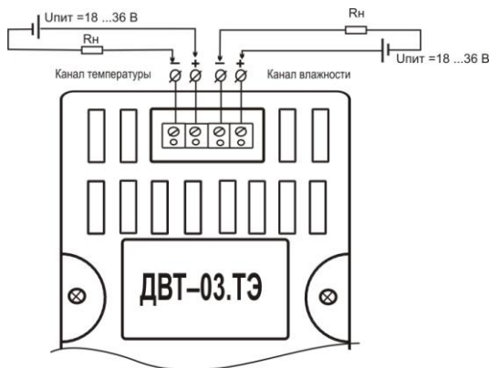
Схема электрическая подключения датчика относительной влажности и температуры ДВТ-03.ТЭ в корпусе на DIN-рейку – D
