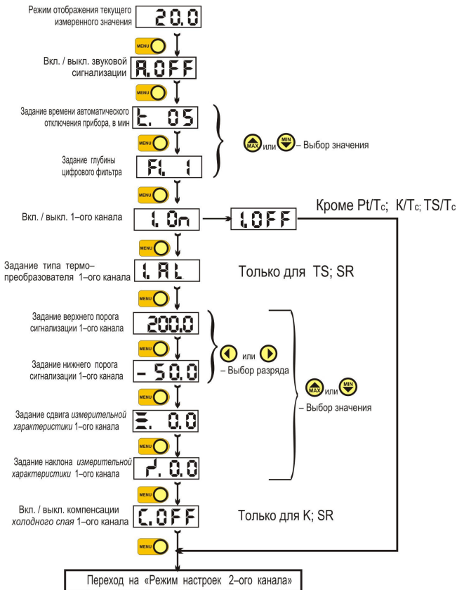
Рисунок 3 – Алгоритм режима настроек прибора IT-8 (Общие настройки и настройки 1-ого канала)
