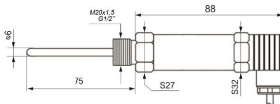
Рисунок 1 – Термопреобразователь с цифровым выходом T.Pt – RS – DIN – 6 – 75 – (-70/+200)
